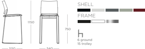
BAR STOOL METAL SLED FRAME KAVBA.PU
