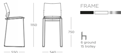
BAR STOOL METAL SLED FRAME KAVBA.U
