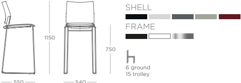
BAR STOOL METAL SLED FRAME KAVBA
